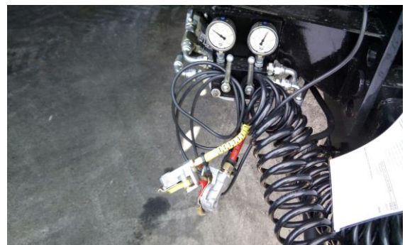
Frein de stationnement pneumatique et freins mixtes (hydrauliques/pneumatiques)
